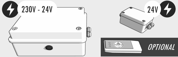
TRANSFORMER BOX AND CONTROL BOX WITH OPTIONAL REMOTE CONTROL / TRANSFORMATORKASTEN UND STEUERUNGSKASTEN MIT OPTIONALER FERNBEDIENUNG / SKRZYŃKA TRANSFORMATOROWA I SKRZYŃKA STEROWANIA Z OPCJONALNYM PILOTEM
