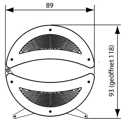
Gerätelänge: 216, alle Maße in cm
