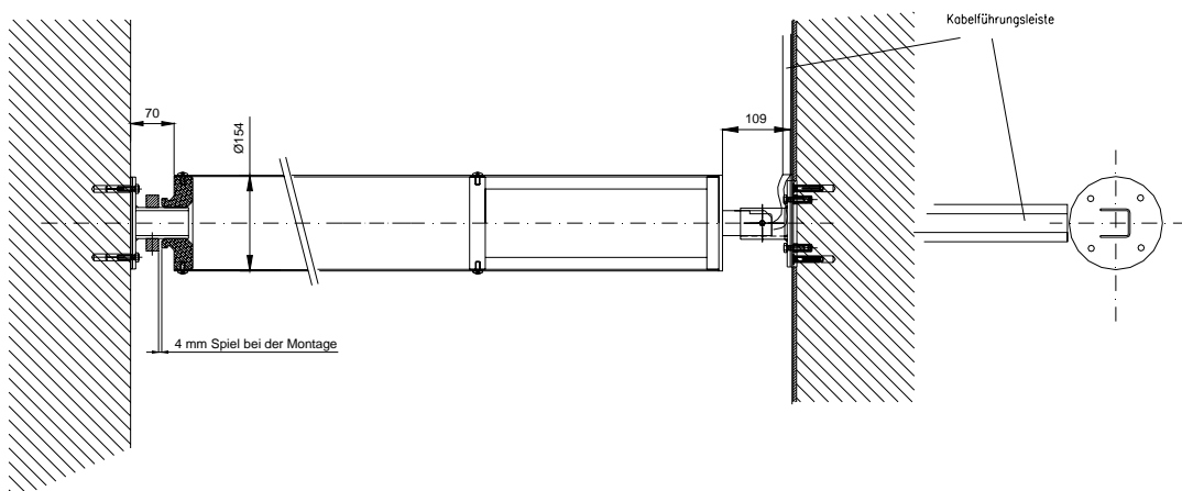
Variante: Folien-/Dünwandbecken
