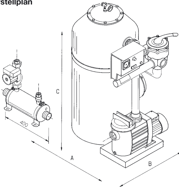
Abbildung: Aufstellplan (Heiz-)Filteranlage
