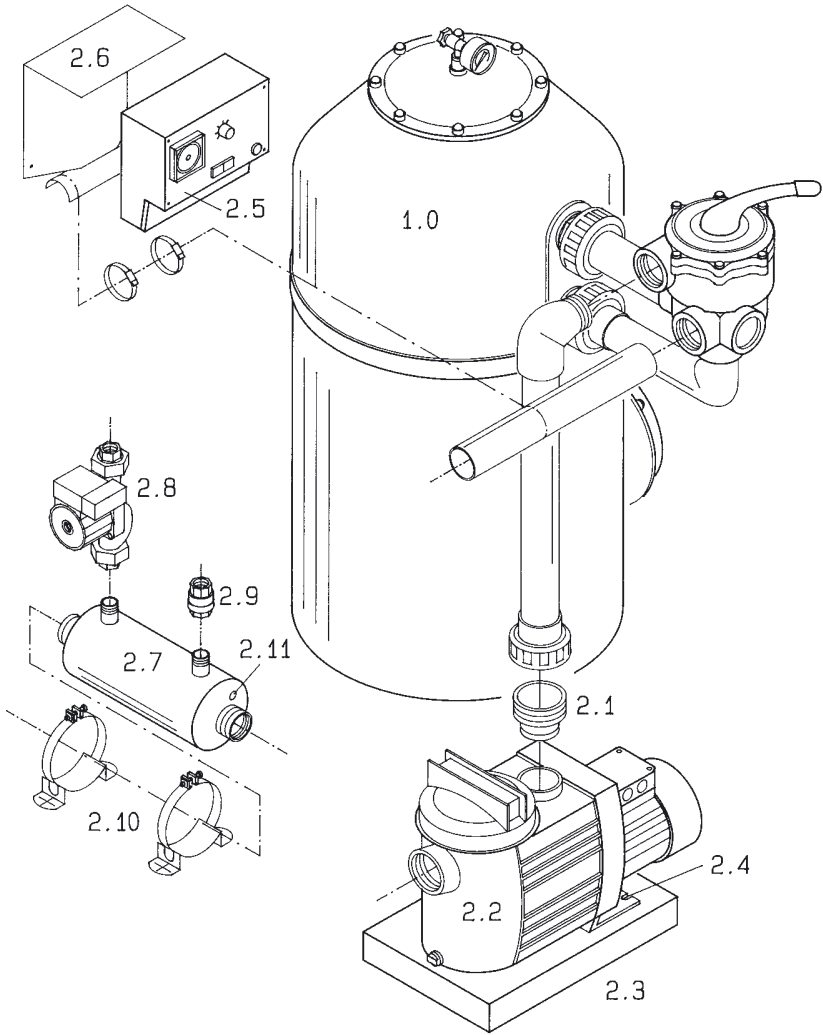
Abbildung: Explosionszeichnung Heiz-Filteranlage
