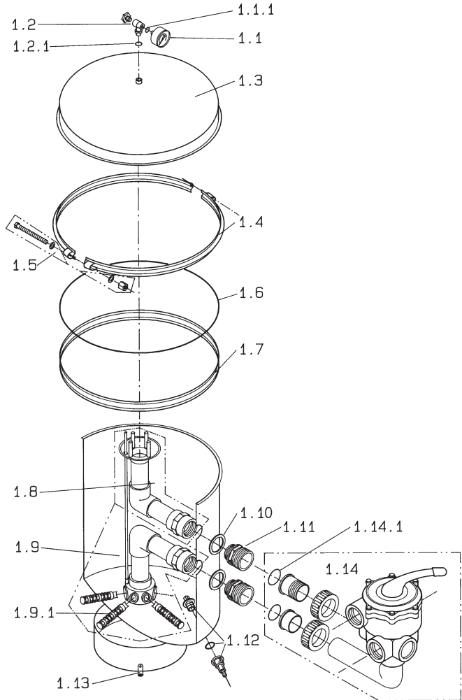
Abbildung: Explosionszeichnung Filterbehälter
