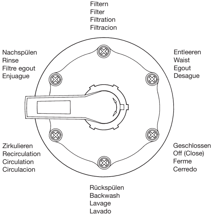
Abbildung: Rückspül-Ventil
