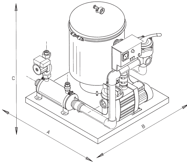
Abbildung: Aufstellplan (Heiz-)Filteranlage
