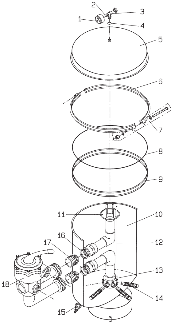
Abbildung: Explosionszeichnung Filterbehälter
