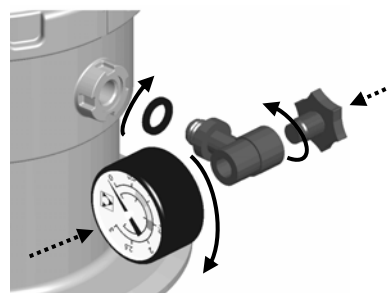
Montage des Manometers (Bei Top-Ventil)
